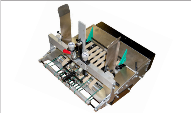
KR 496 FEXW – Profi Friction Feeder Für eine einfache Zuführung schwieriger Materialien. Flexibel kombinierbar mit dem Vakuum Transport Basen von Kirk-Rudy™.
